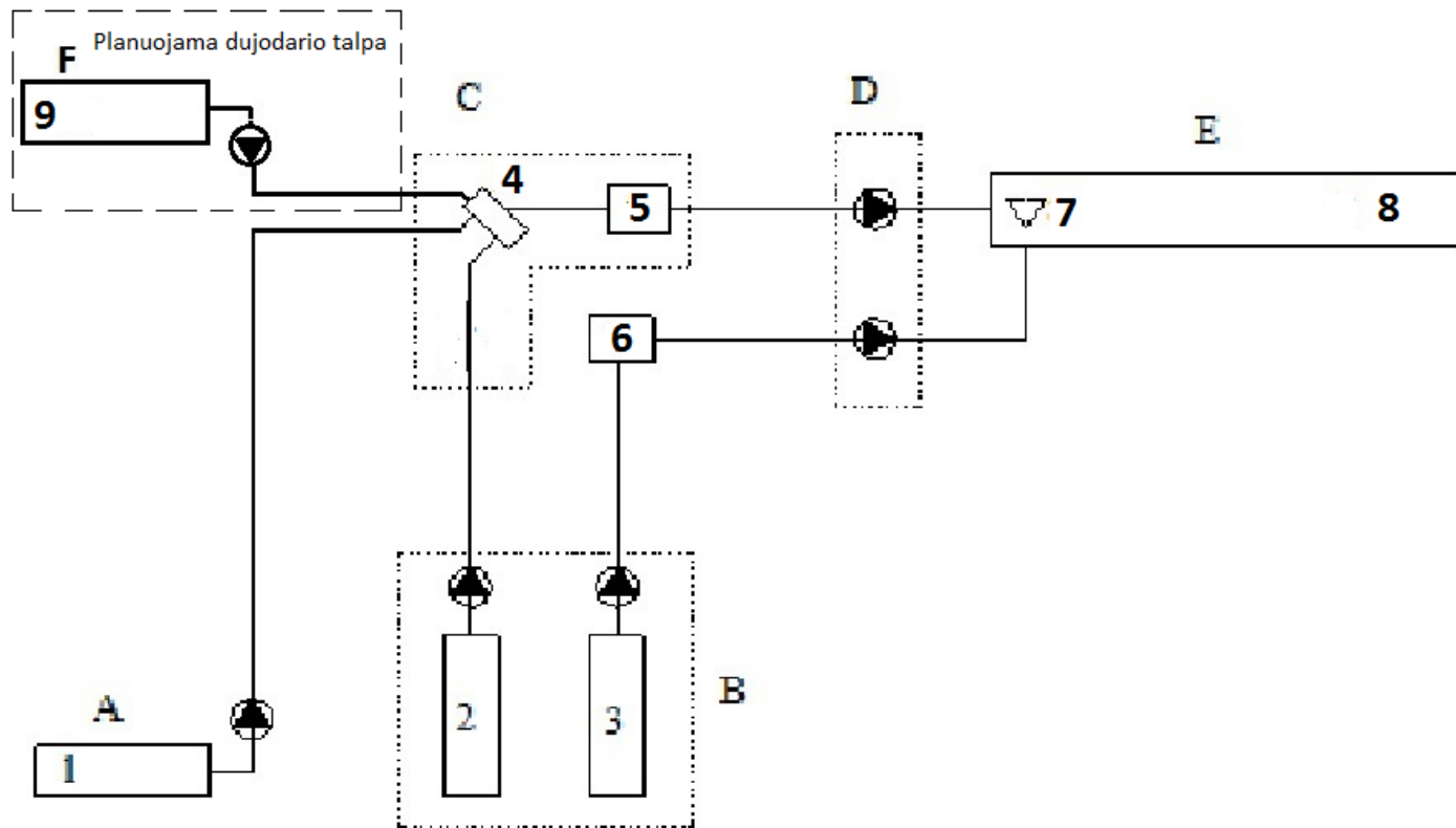
4 pav. Plokščių liejimo technologinio proceso schema
