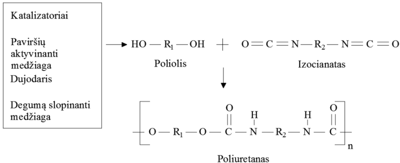
3 pav. Klasikinė Struktūrinė poliuretano putų sintezės schema 3
